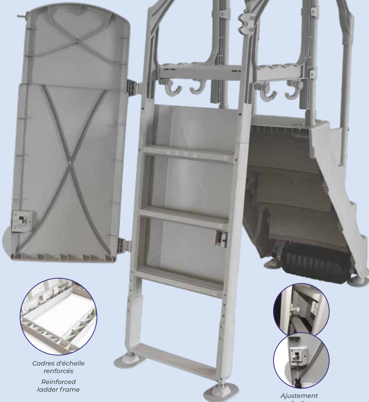
Charnières à ressort Spring hinges
